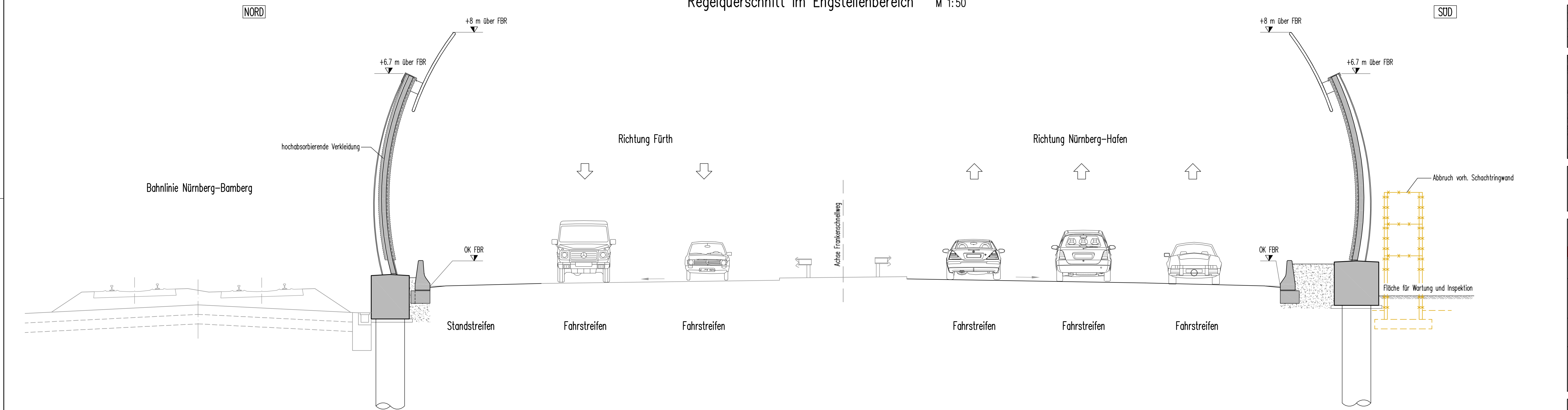
Regelquerschnitt im Engstellenbereich M 1:50
